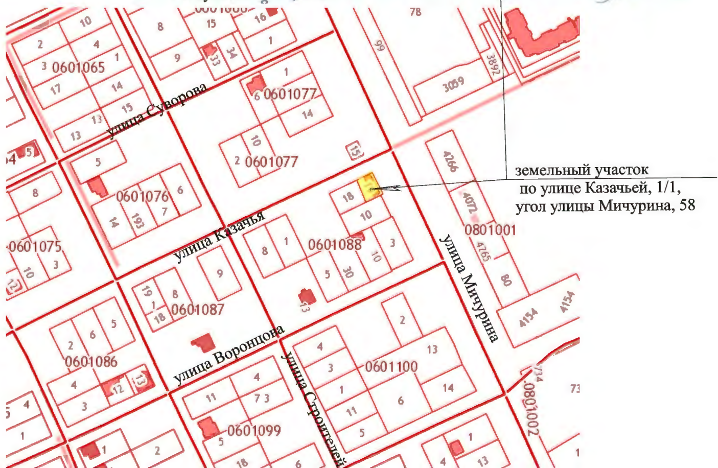
Ситуационный план
