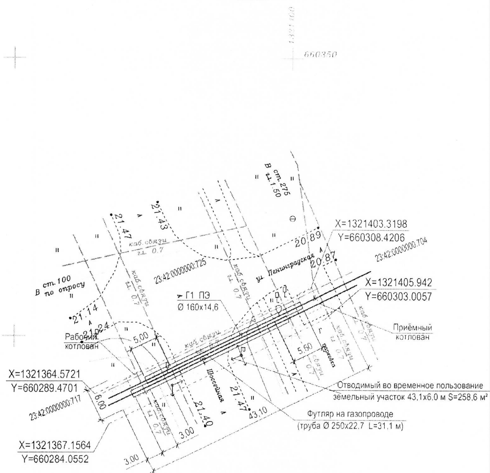
План земельного участка с границами публичного сервитута М 1:500
